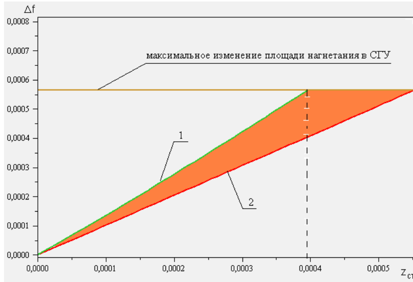
Рис. 7. Изменение площади нагнетания в СГУ: 1 — с учетом взаимодействия прямых и обратных потоков в СГУ; 2 — без учета взаимодействия прямых и обратных потоков в СГУ
