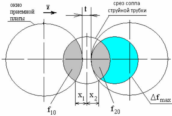
Рис. 3. Рабочие площади струйного гидрораспределителя
