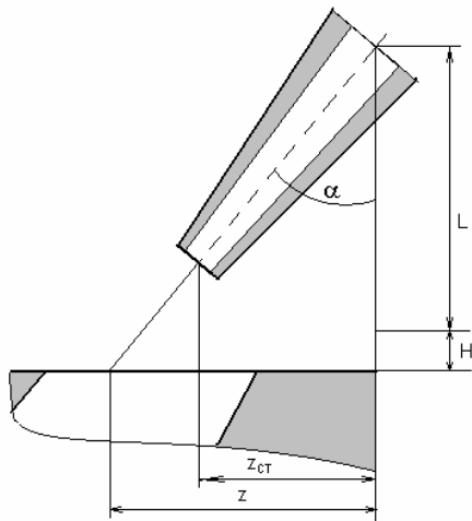
Рис. 5. Схема смещения струйной трубки
