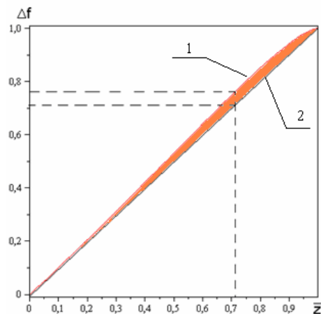
Рис. 4. Безразмерное изменение площади нагнетания в СГУ: 1 — нелинейная зависимость; 2 — линейная зависимость
