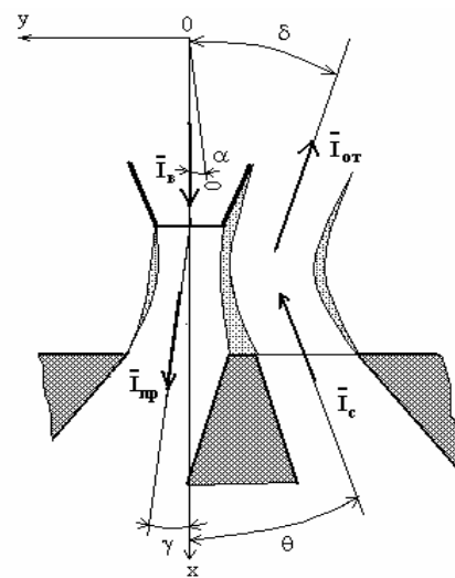
Рис. 6. Схема взаимодействия струй жидкости в СГР
