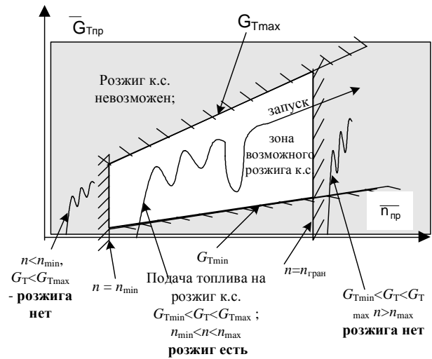
Рис. 3. Области розжига при запуске
