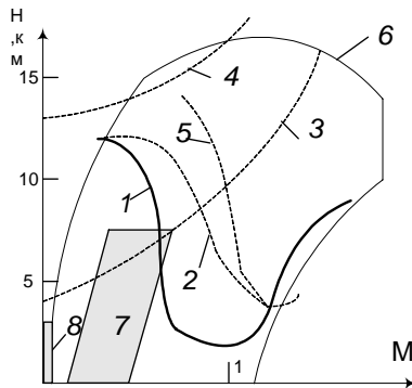
Рис. 4. Границы возможного запуска КС по высоте и скорости полета на примере одновального ТРД ( \pi_{к.расч.}^* = 4,5 )
