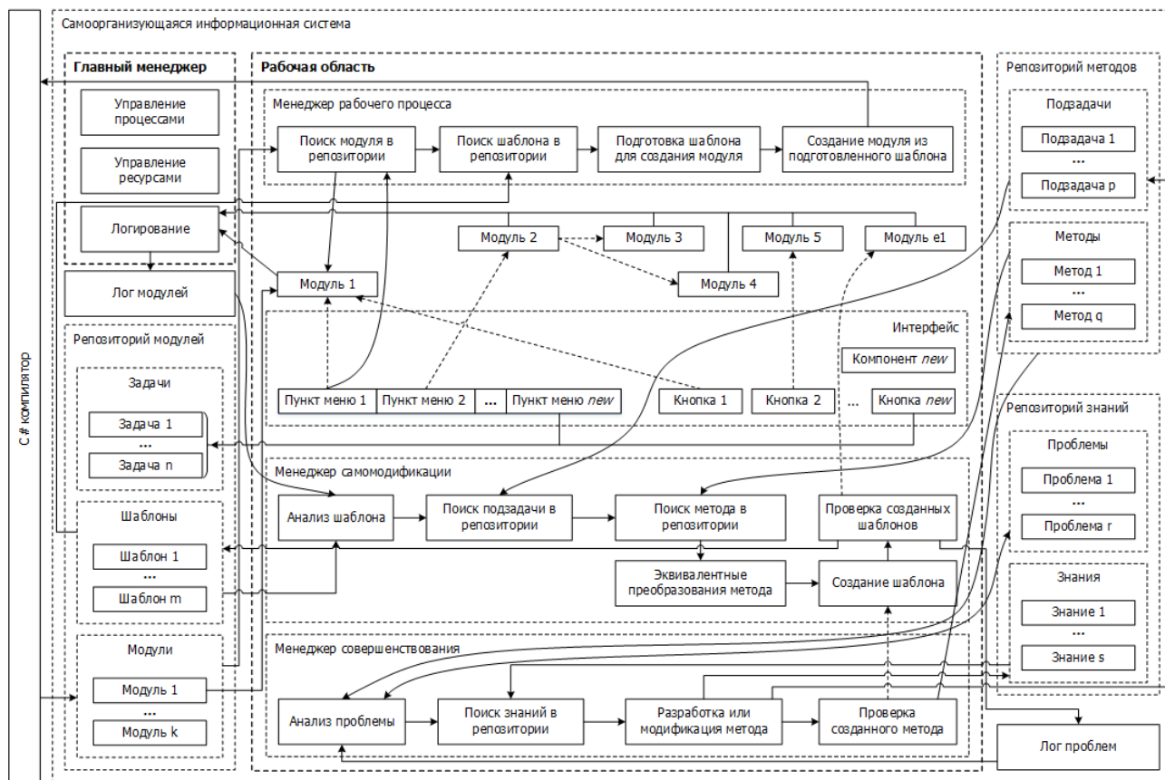
Рис. 3. Физическая модель эффективной организации вычислительного процесса в СИС.
