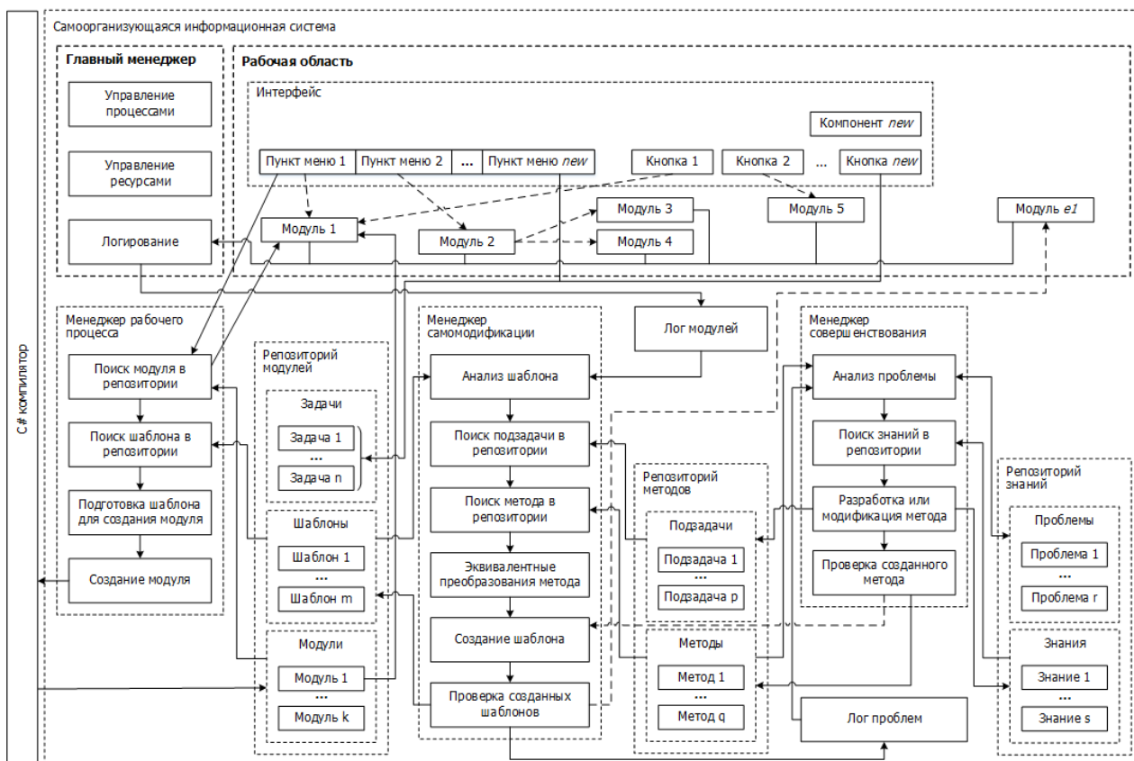
Рис. 2. Физическая модель организации вычислительного процесса в СИС
