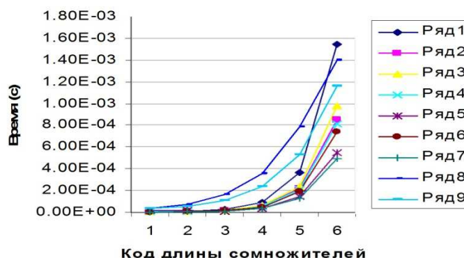
Графики зависимостей времени вычислений от длины сомножителей
