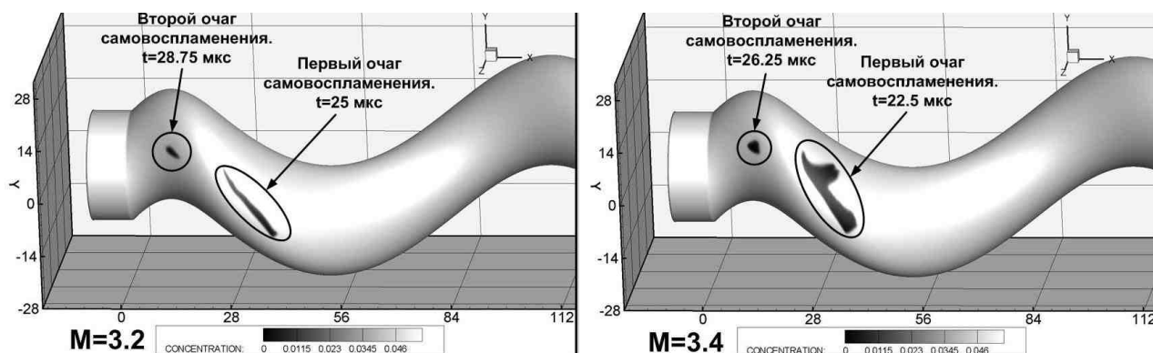
Рис. 6. Возникновение очагов самовоспламенения смеси для случаев перехода ударной волны в детонационную. Поле концентрации пропана на поверхности трубы
