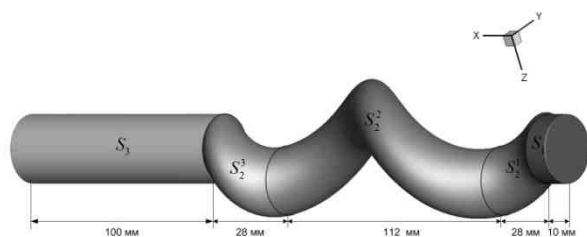
Рис. 5. Схема винтовой трубы
