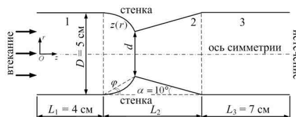
Рис. 3. Схема профилированной трубы с параболическим сужением и коническим расширением
